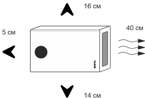
Горизонтальное расположение, выход воздушного потока справа
