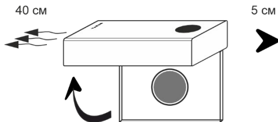
Горизонтальное расположение Выход воздушного потока слева
