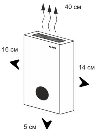
Вертикальное расположение, выход воздушного потока сверху
